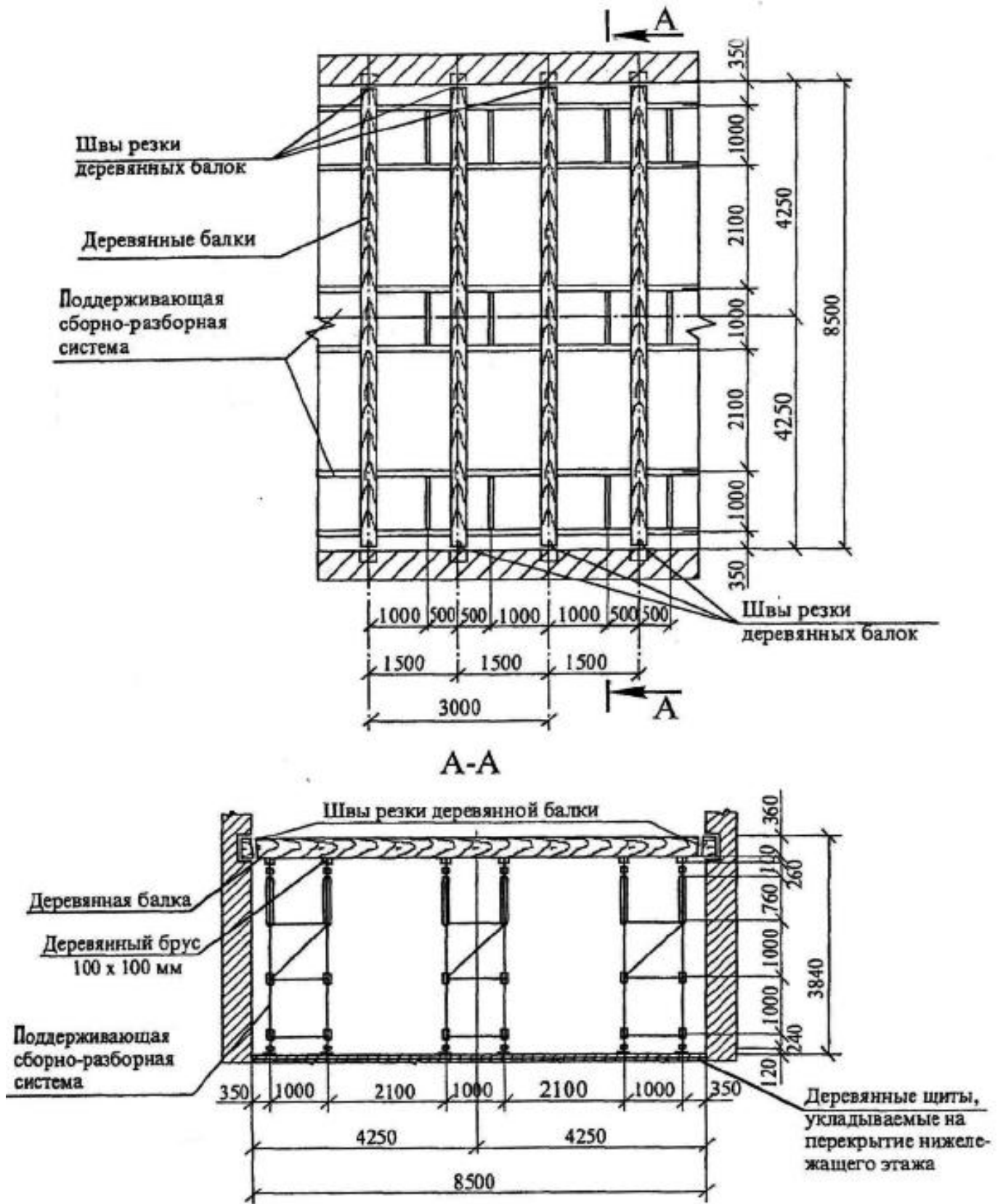
Рисунок 2 - Схема разборки междуэтажного перекрытия по деревянным балкам
